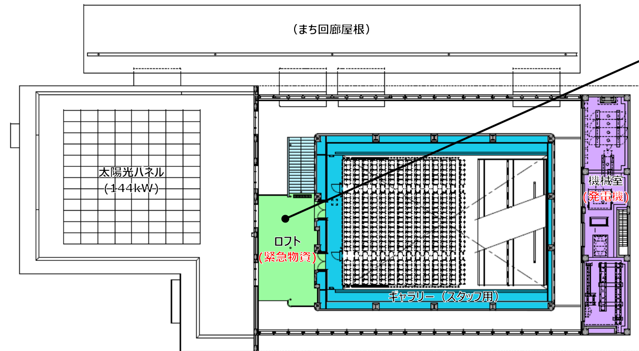
〔2階平面図〕
