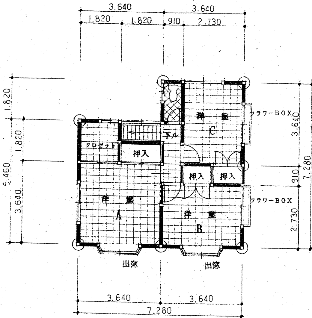
2 階 平 面 図 1:100
