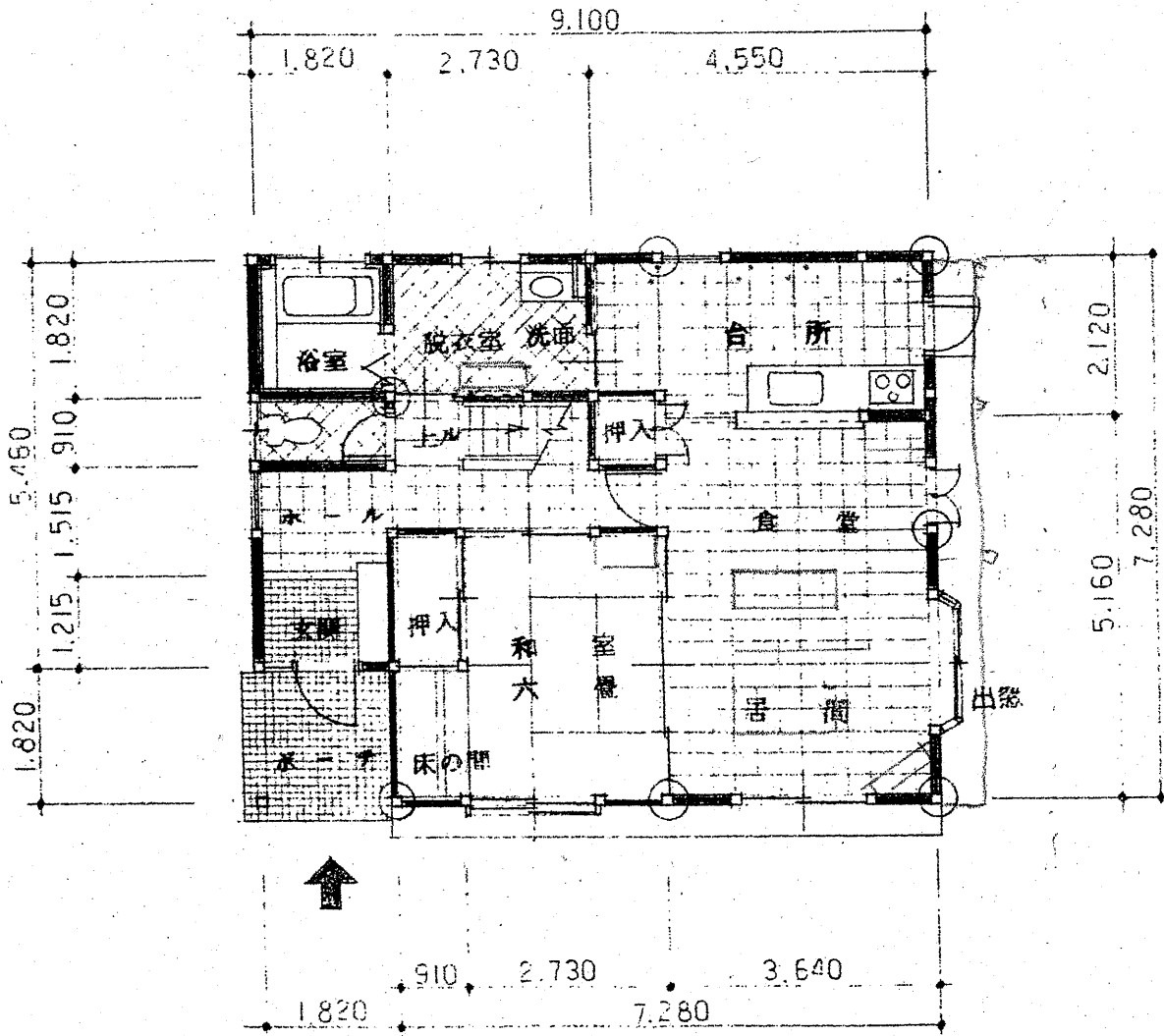
1 階 平 面 図 1:100
