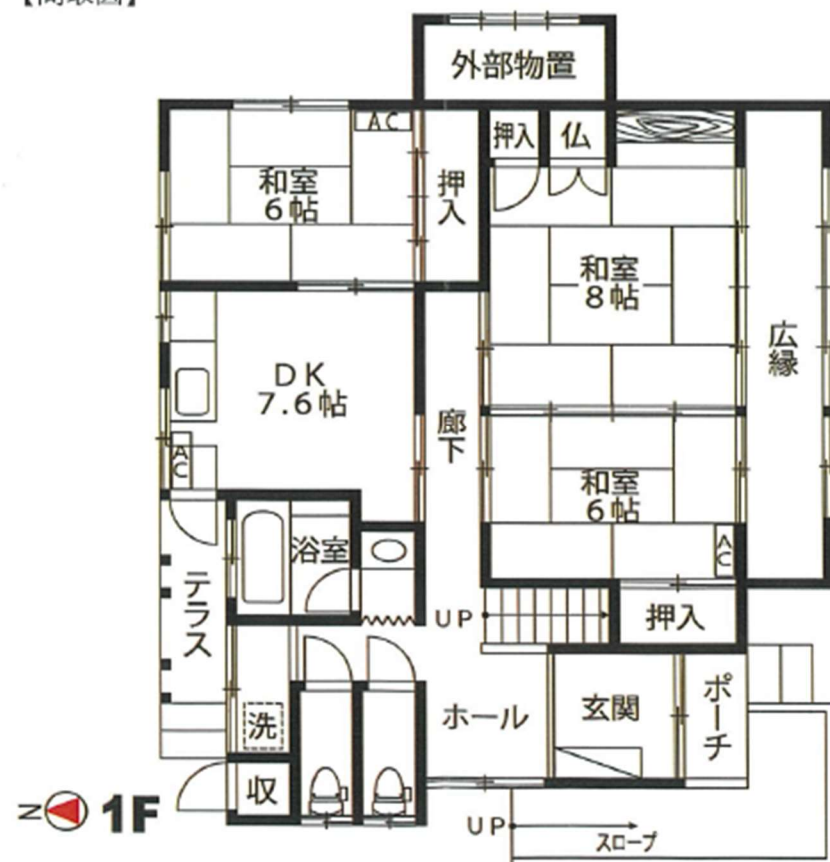
【間取図】
