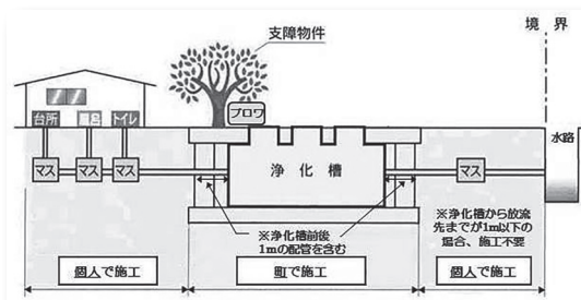
浄化槽図（水路）
