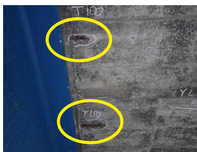
床版下面の鉄筋露出 (供用 48 年)
